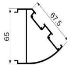
JY-75ZD-09 corner Weight : 1.135 kg/m
