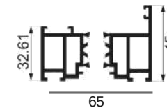
JY75ZD-21 + JY75ZD-20 door frame Weight : 0.88 kg/m , 0.57 kg/m
