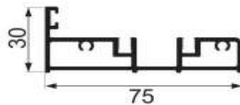
JY-75ZD-39 bottom rail Weight : 1.16 kg/m
