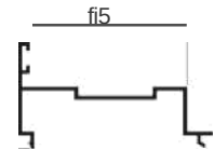
JY-75ZD-04 door frame closing Weight : 0.46 kg/m
