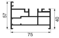
JY-75ZD-17 side frame Weight : 2.01 kg/m
