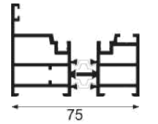
JY75ZD-38 + JY75ZD-37 side frame Weight : 1.19 kg/m , 0.95 kg/m
