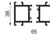
JY-75ZD-22 center column Weight : 0.90 kg/m
