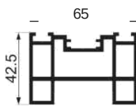
JY-75ZD-27 door frame Weight : 1.98 kg/m
